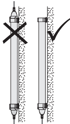
Vertikale Montage
