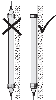
Montaje vertical
